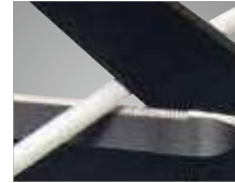
Haltekerben am Beginn der Schneide für Drähte und runde Materialien
